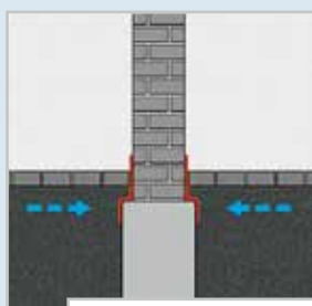
Fundamentabdichtung
