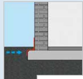
Sockelabdichtung
